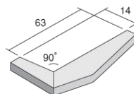
90° 曲り (接着)
